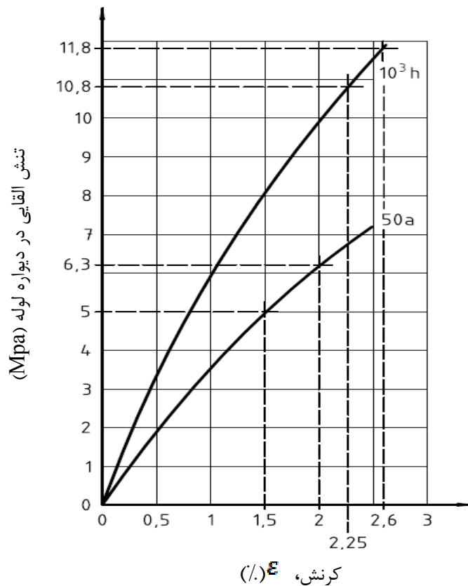
نمودار الف-۱- نمودار تنش-کرنش هم‌زمان برای PP-H در دمای ۲۰ °C
