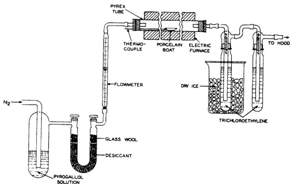
شکل یک- دستگاه اندازه گیری دوده
